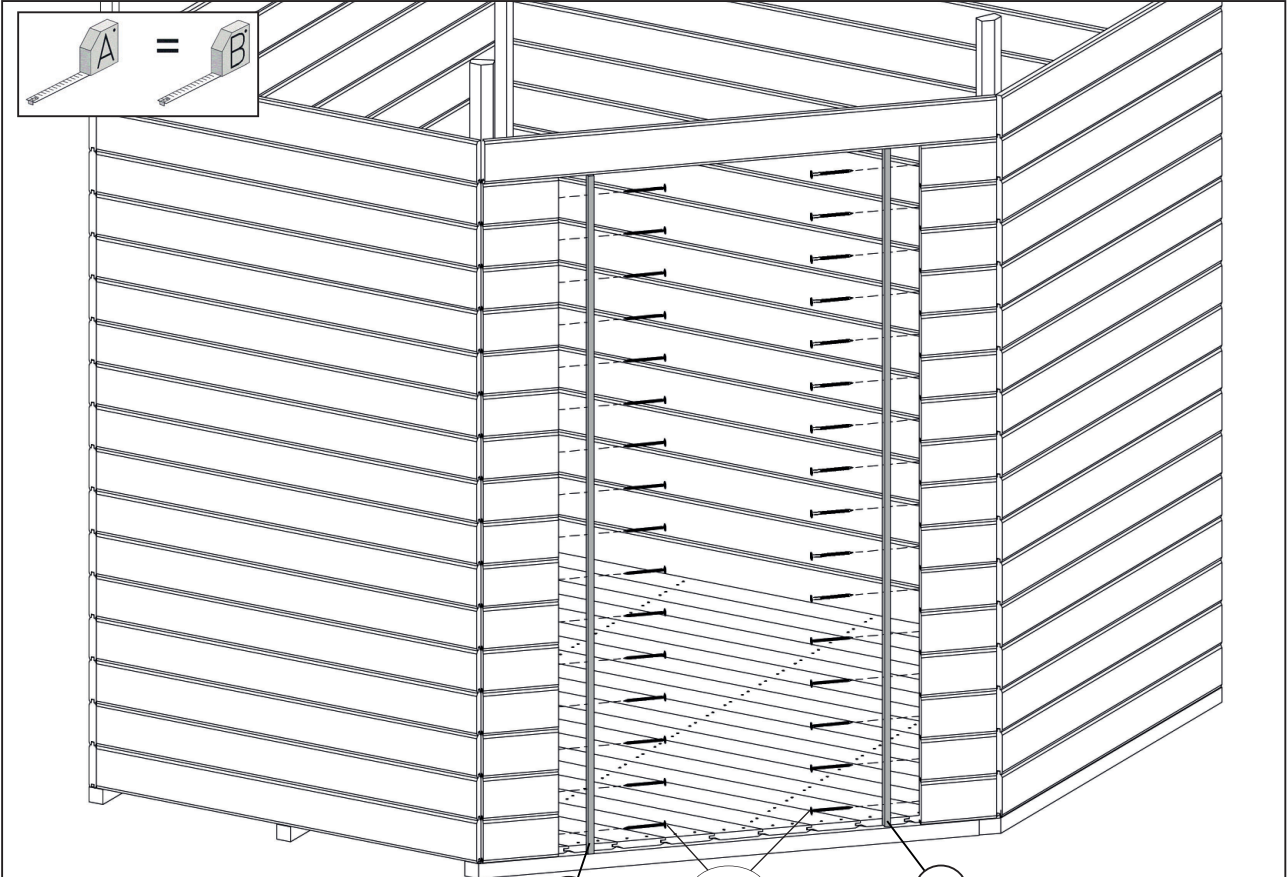
Abbildung Art.-Nr.: 229.2121.1X400 (34) 16x M2 (34)
